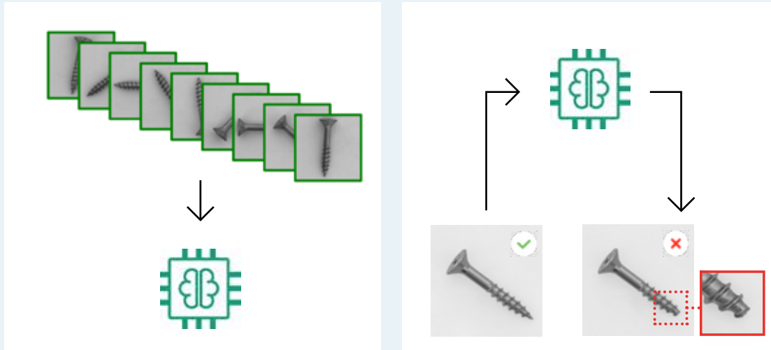
Aus Bildern von intakten Schrauben lernt der Algorithmus, wie eine intakte Schraube aussieht (links). Auf Basis dieses Wissens werden Schrauben mit Fehlern erkannt (rechts).
